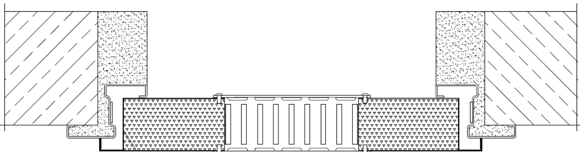
Przekrój poziomy drzwi z kratką
